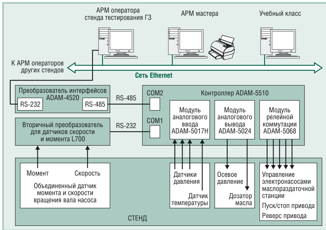
Рис. 5. Функциональная схема системы управления стендом
